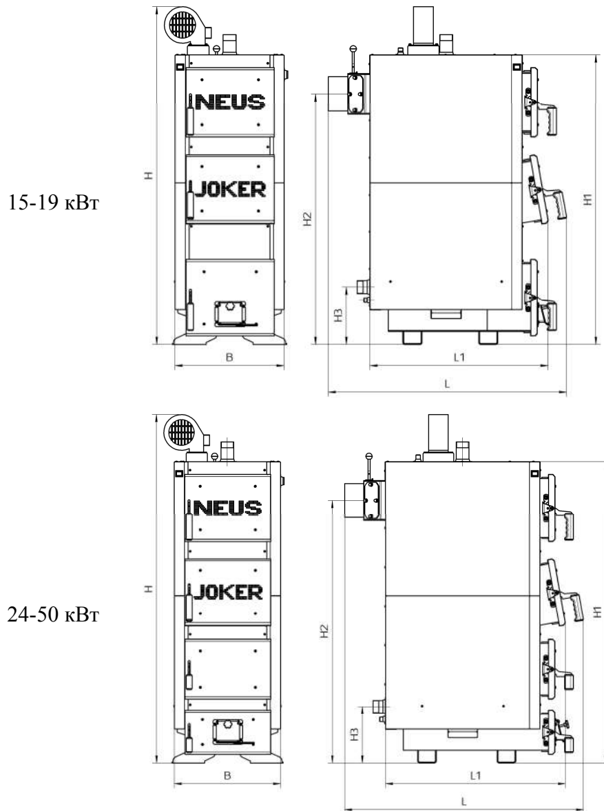
Рисунок 1 – Габаритне креслення котла NEUS JOKER (NEUS JOKER-Плюс)
