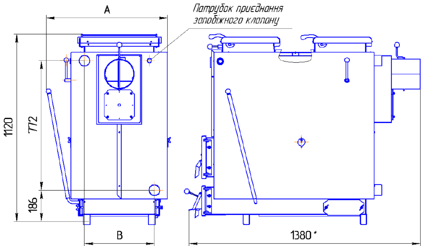
Рисунок 2. Приєднувальні розміри
