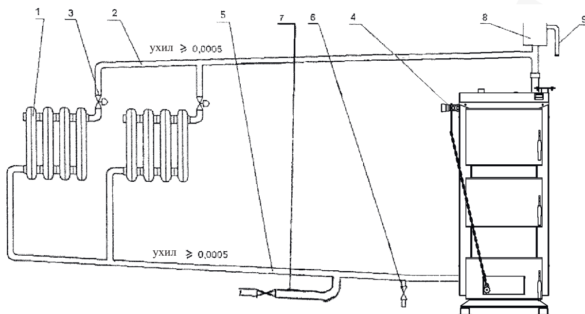
Мал. 3. Схема під'єднання котла до системи опалення.
