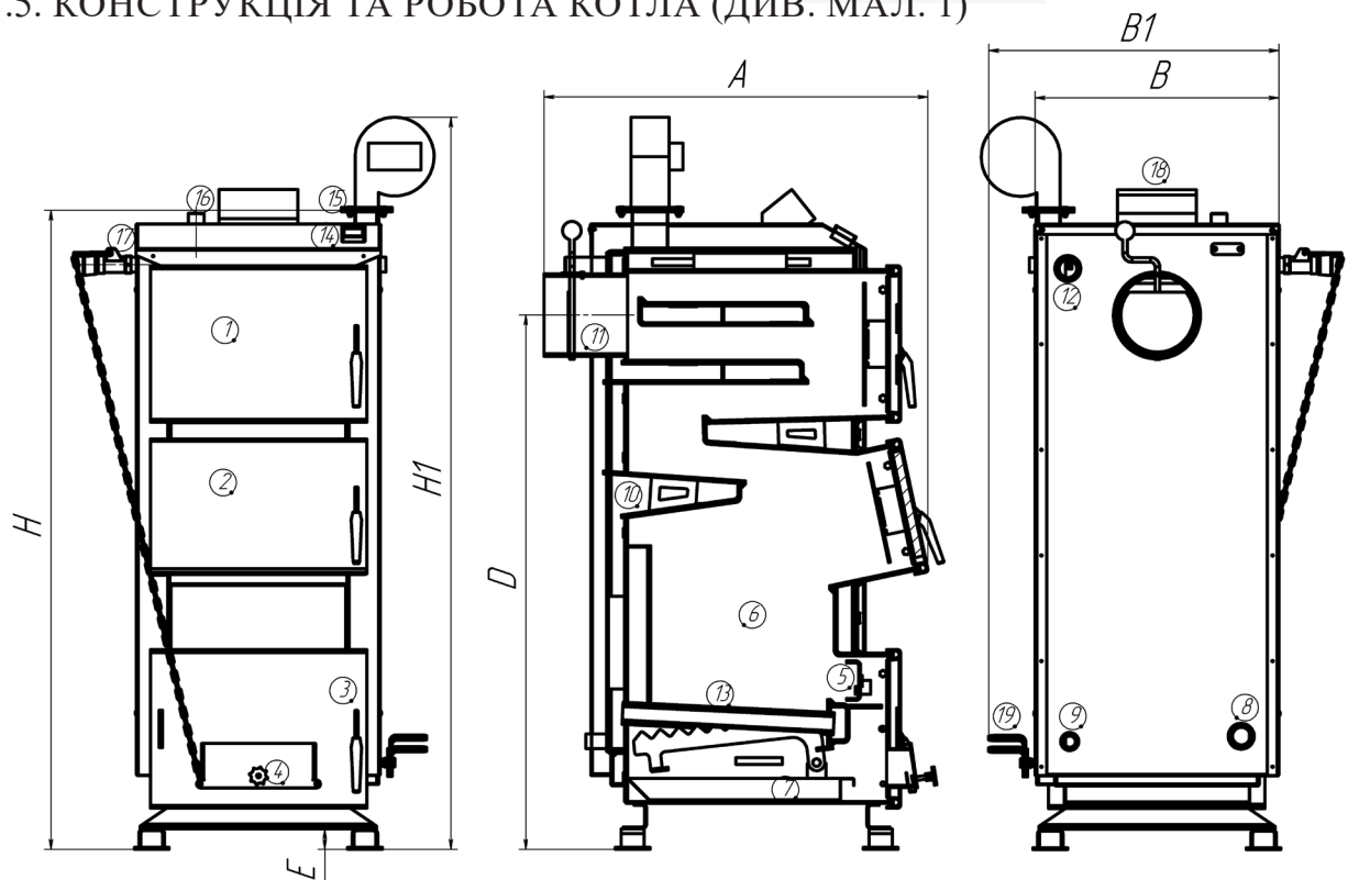
Мал.1. Загальний вигляд котла Thermo Alliance Vulcan PLUS і його конструкція
